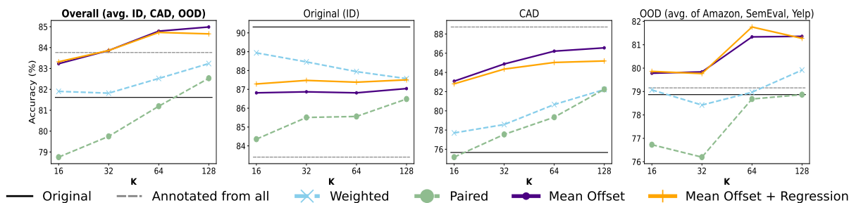
Fig. 7: SMPNet
