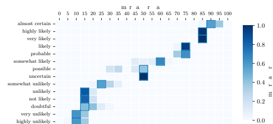
(f) GPT-4o
