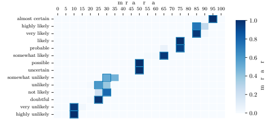
(h) GPT-4
