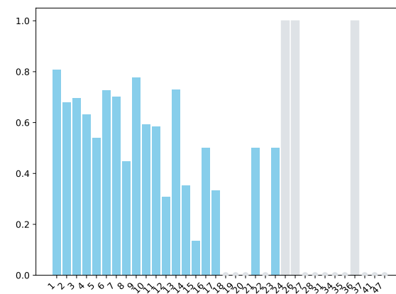
(d) Senseval2
