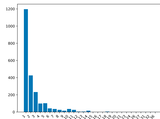
(d) Senseval2
