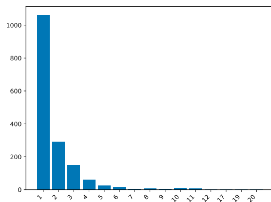
(b) SemEval2013
