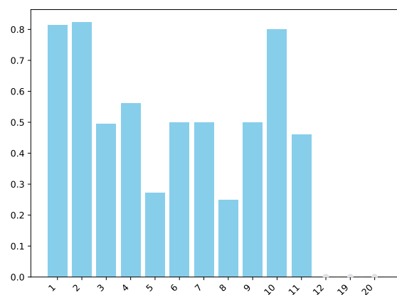
(b) SemEval2013
