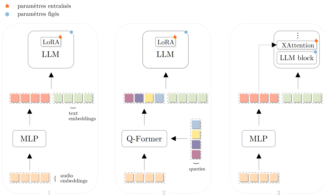
FIGURE 1 – Trois architectures pour intégrer des informations audio dans un modèle de langage : (1) les représentations audio sont simplement passées en tant que préfixe du LLM ; (2) les embeddings sont projetés via un module Q-Former composé de queries apprenables ; (3) les représentations audio et textuelles sont fusionnées à l’aide d’un mécanisme de cross-attention. Par ailleurs, le MLP d’entrée peut être étendu et, si nécessaire, intégrer des couches d’attention.
