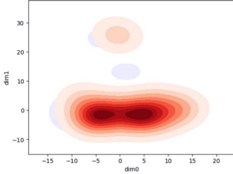
FIGURE 1 – Couverture des plongements lexicaux d’entrée (bleu) et de sortie (rouge) après une réduction de dimension par ACP (Analyse en Composantes Principales - PCA pour Principal Component Analysis). Les zones violettes représentent le contenu de l’entrée, tandis que les zones rouges correspondent à la sortie. Les zones bleues non couvertes indiquent des informations manquantes ou insuffisamment représentées, signalant ainsi des omissions.
