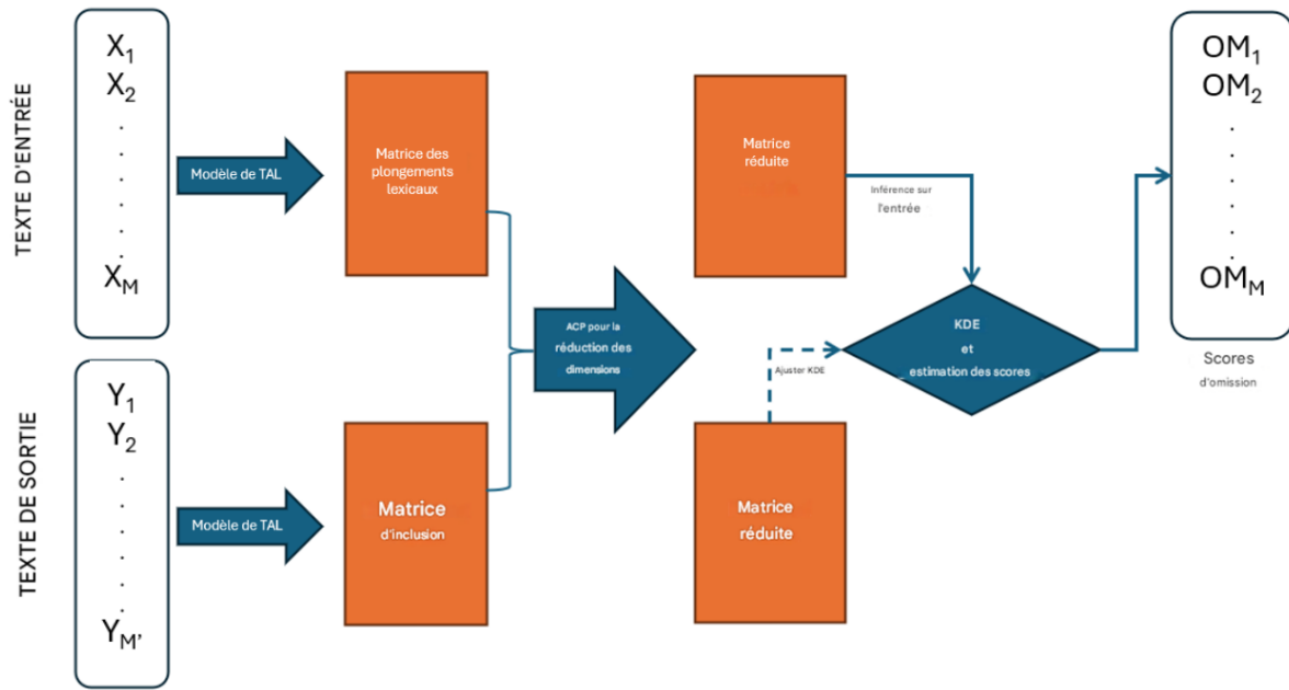
FIGURE 2 – Vue d'ensemble de la détection d'omission utilisant KDE.
