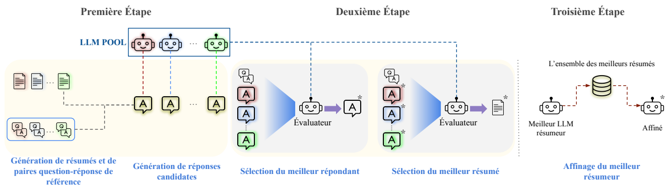
FIGURE 1 – Un aperçu de QUARTZ pour le résumé non supervisé de dialogues orienté tâche.
