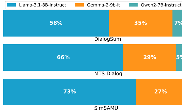
FIGURE 3 – Taux de victoire des LLMs sur les jeux de données.
