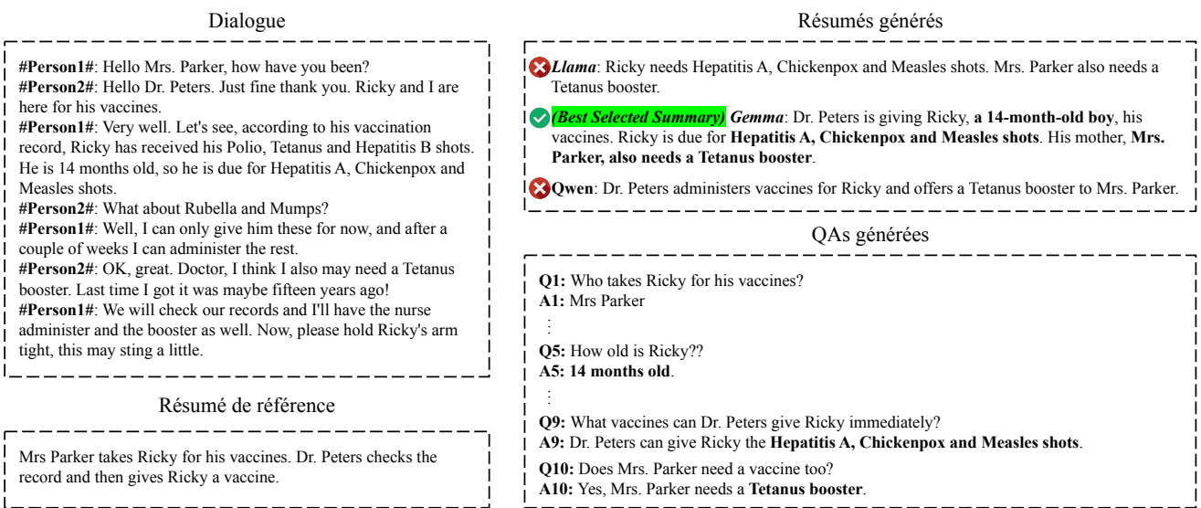
FIGURE 4 – Exemple de dialogue du jeu de données DialogSum. Gauche : Dialogue original et résumé de référence. Droite : Résumés générés par chaque LLM du pool, accompagnés des questions-réponses liées à la tâche. Les informations supplémentaires introduites par le meilleur résumé sélectionné sont mises en gras .
