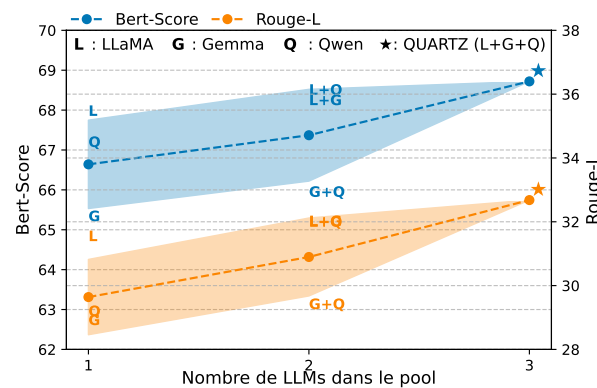
FIGURE 2 – Impact de la taille du pool de LLM sur la performance, avec moyenne ( pointillés ) et écart-type ( ombré ) (voir Annexe A.1).
