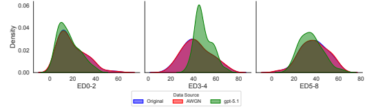
(a) GPT-5.1 - 2020
