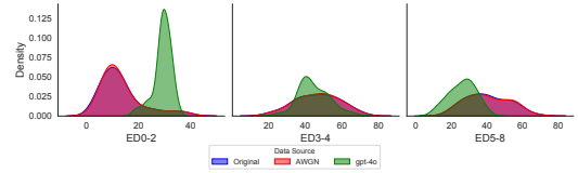
(d) GPT-4o - 2023
