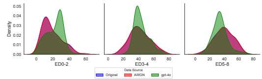
(b) GPT-4o - 2021
