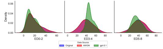
(d) GPT-5.1 - 2023
