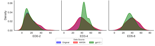
(b) GPT-5.1 - 2021
