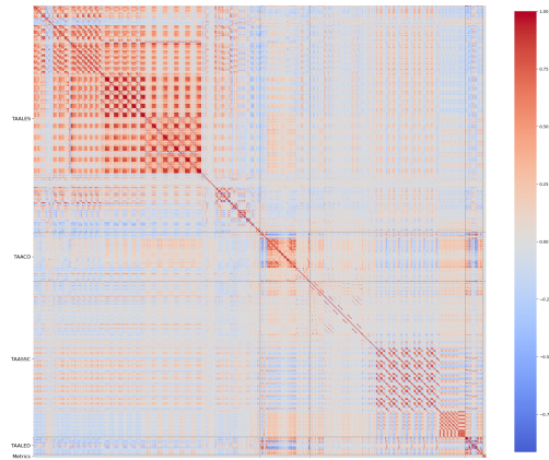
(d) Simple side of D-Wikipedia (document-level).
